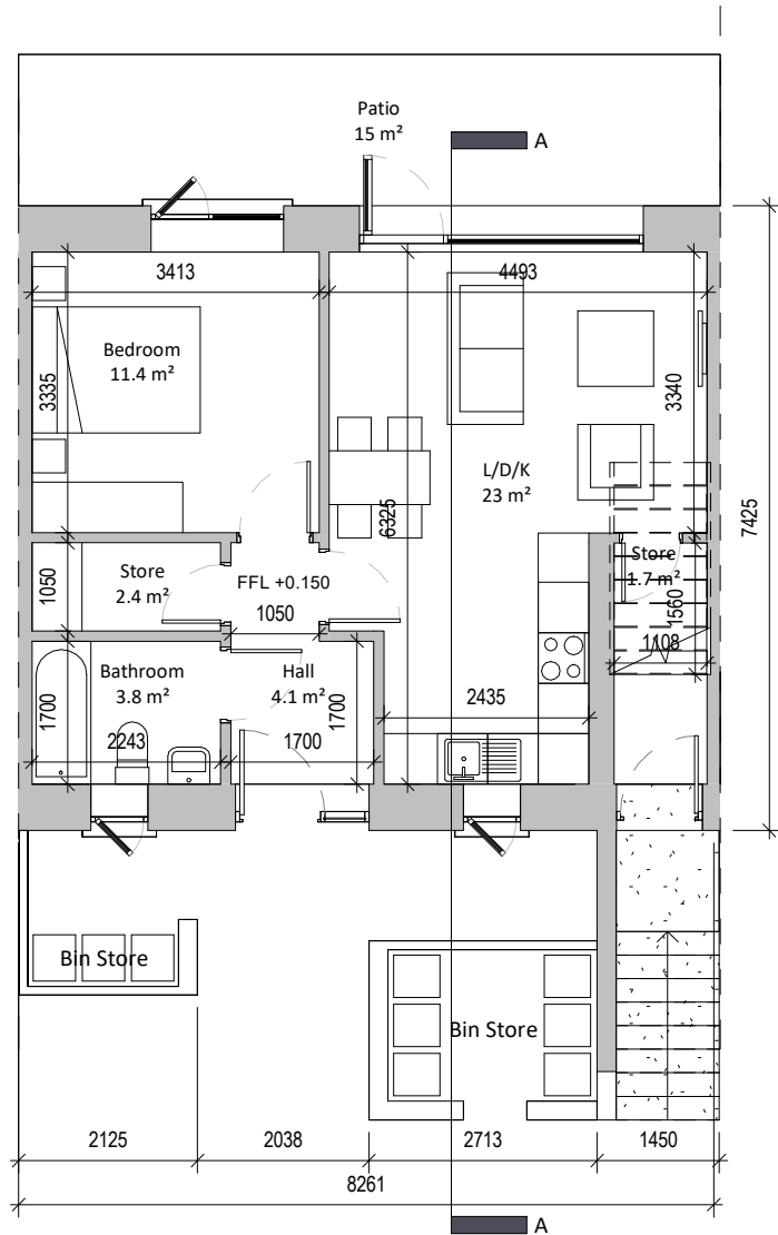
① Ground Floor (Simplex 1A) 1 : 100
