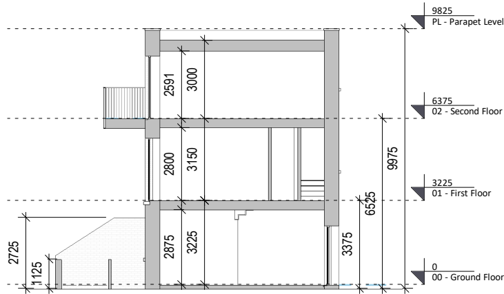
4 Section A-A 1 : 200
