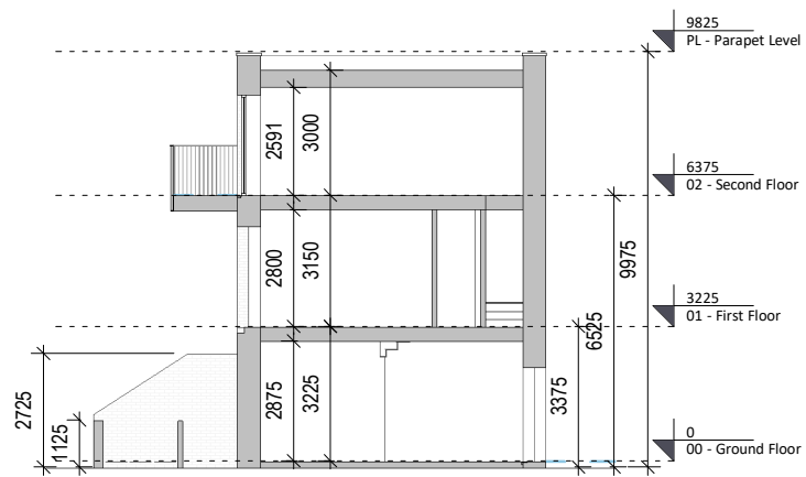
4 Section A-A 1 : 200
