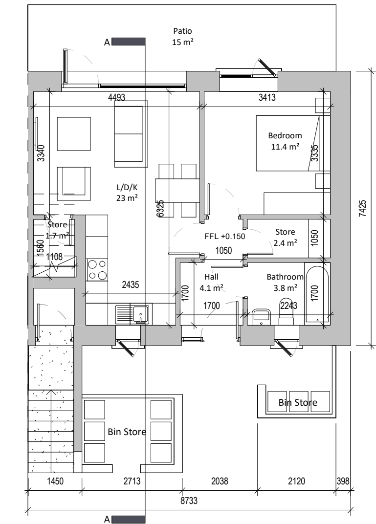
① Ground Floor (Simplex 1R1A) 1 : 100
