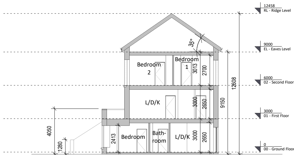
4 Section A-A 1 : 200
