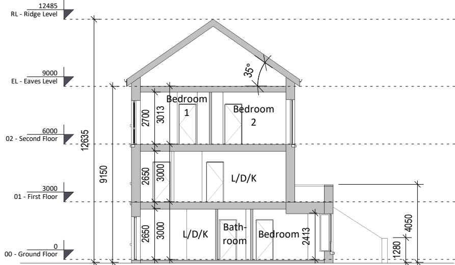
4 Section A-A 1 : 200
