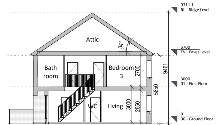
5 Section A-A 1 : 200
