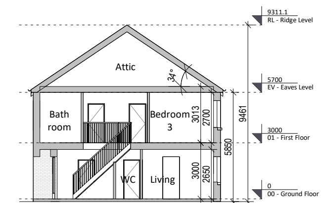
6 Section A-A 1 : 200
