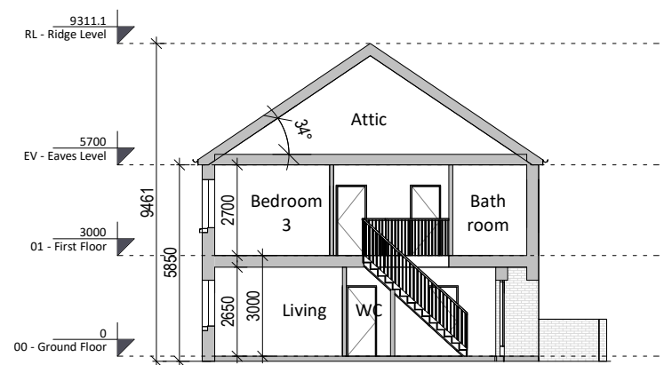
5 Section A-A 1 : 200
