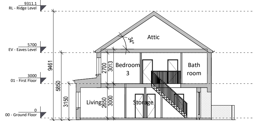
5 Section A-A 1 : 200
