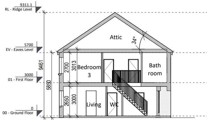
6 Section A-A 1 : 200
