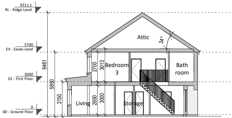
⑥ Section A-A 1 : 200
