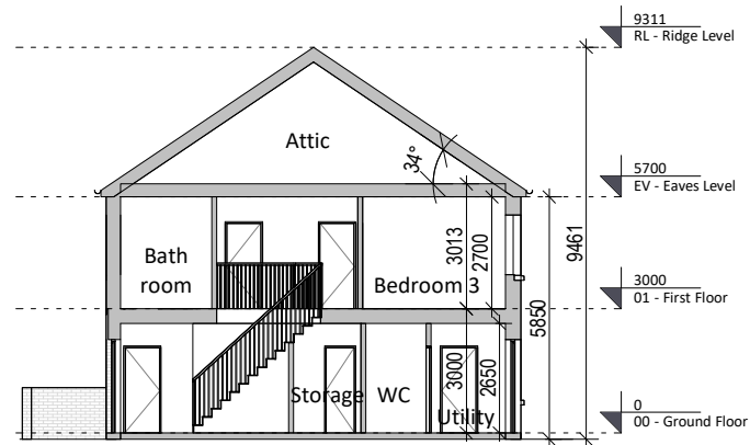
5 Section A-A 1 : 200
