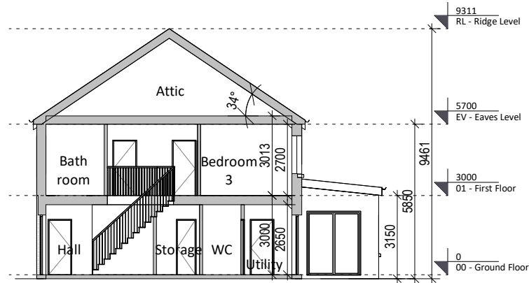
⑥ Section A-A 1 : 200
