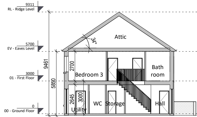
5 Section A-A 1 : 200
