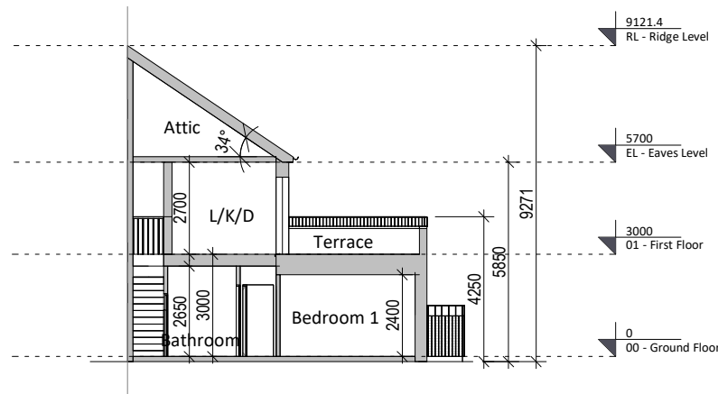
⑥ Section A-A 1 : 200
